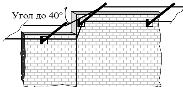
Рисунок 2.3 – Крепление КМЧ и проводов при перепадах высоты
